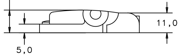
Vorderansicht front view
