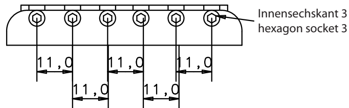
Vorderansicht front view
