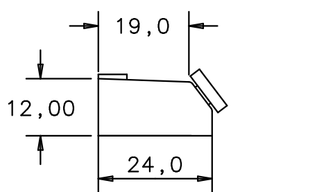
Seitenansicht side view
