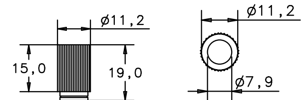
Einschlagmutter insert
