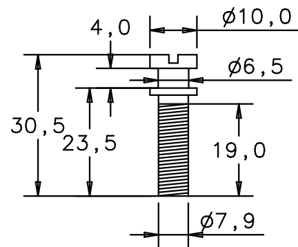
Höhenverstellerschraube level adjustable screw
