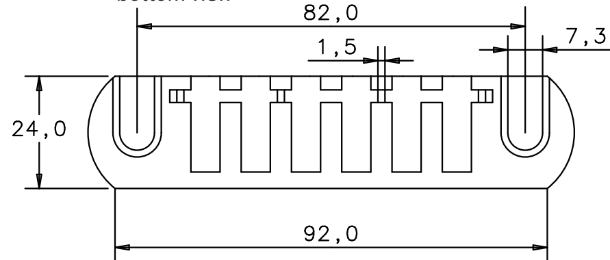
Untersicht bottom view
