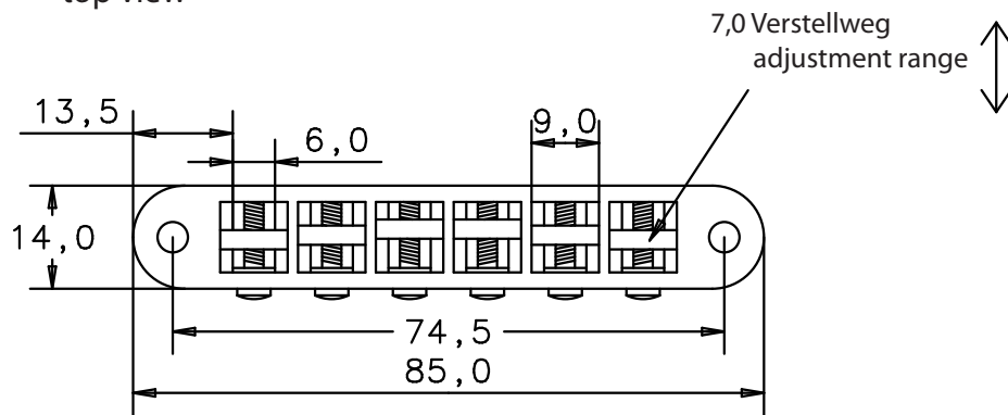
Draufsicht top view
