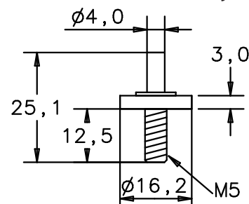
Höhenverstellschraube level adjustable screw
