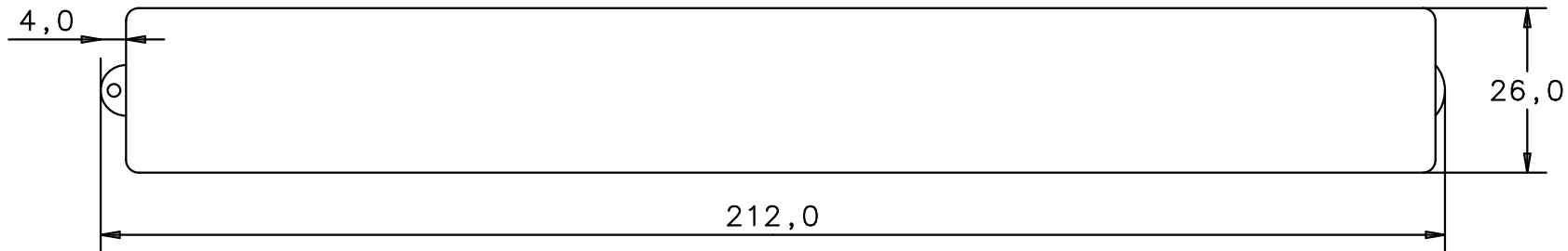
Untersicht bottom view
