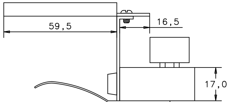
Seitenansicht von links side view left
