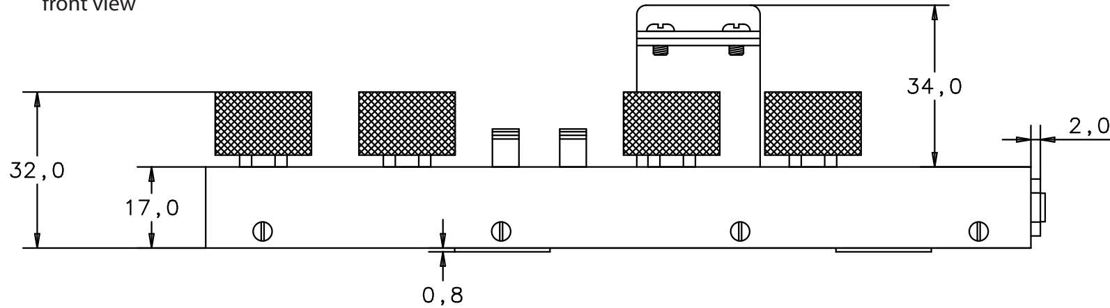
Vorderansicht front view
