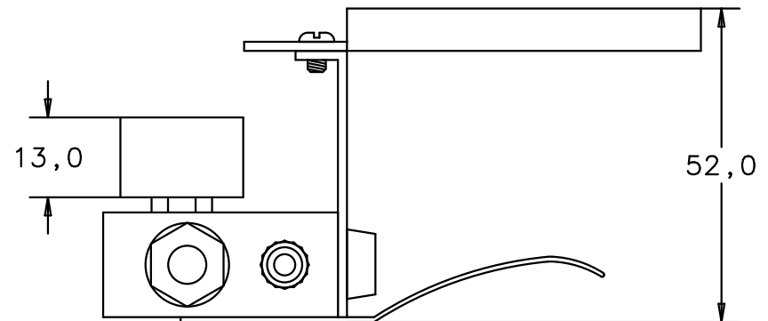
Seitenansicht von rechts side view right
