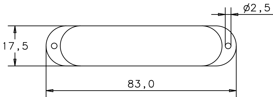
Draufsicht top view
