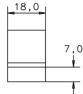
Seitenansicht von rechts side view right
