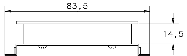
Rückansicht back view
