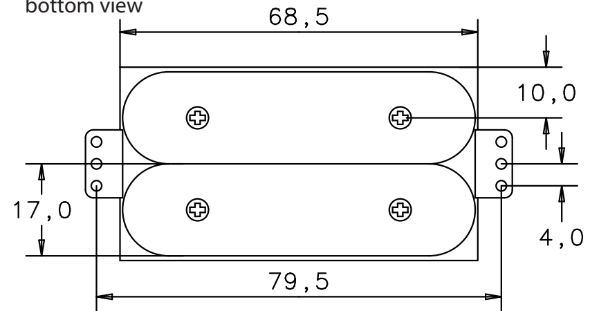
Unteransicht bottom view
