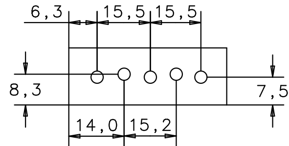
Untersicht bottom view
