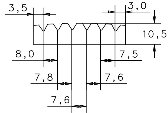
Rückansicht back view
