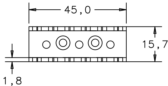
Draufsicht top view
