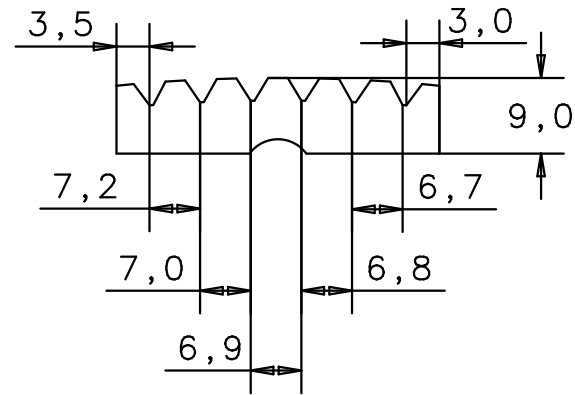
Rückansicht back view
