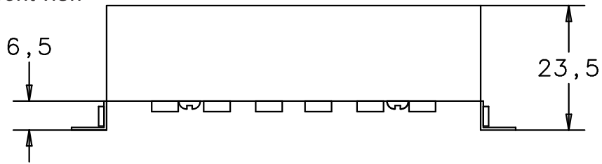
Draufsicht top view
