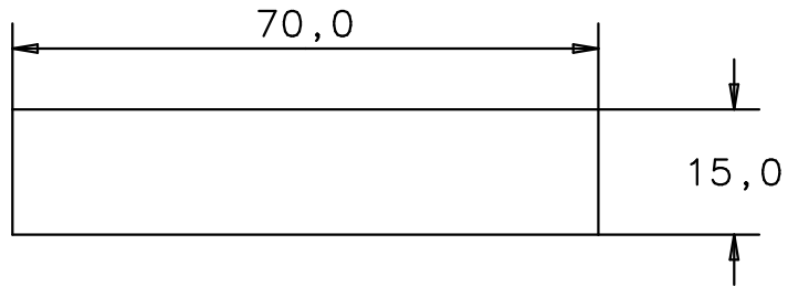
Vorderansicht front view
