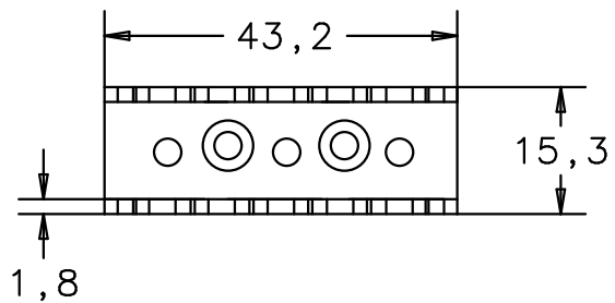
Draufsicht top view
