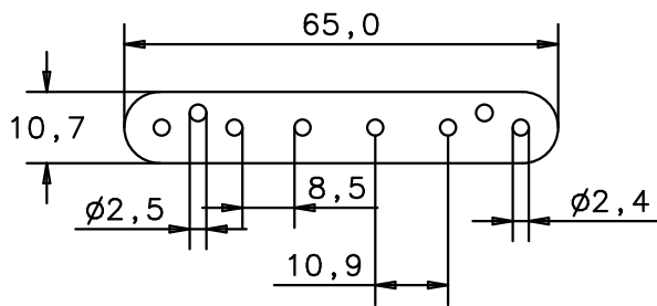
Untersicht bottom view
