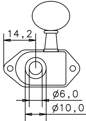
Seitenansicht von links side view left
