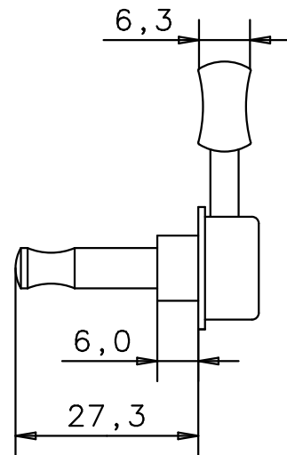
Seitenansicht von links side view left
